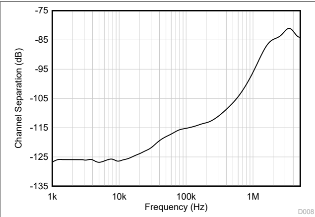
图 6-37. 通道隔离与频率间的关系
