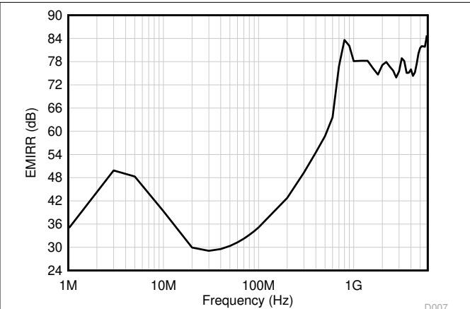
图 6-38. EMIRR ( 电磁干扰抑制比 ) 与频率间的关系
