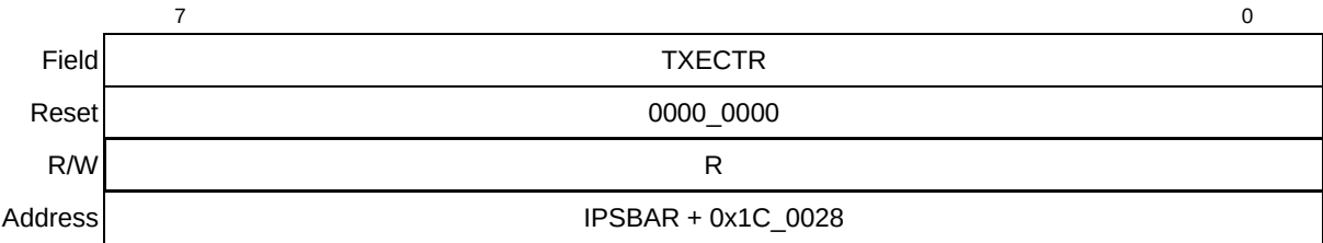
Figure 25-17. FlexCAN Transmit Error Counter (TXECTR)
